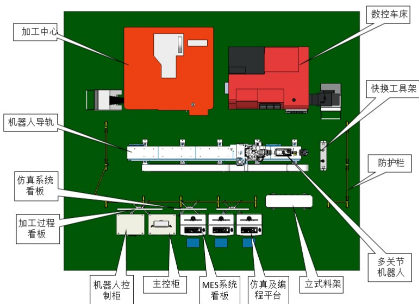
图 1 切削加工智能制造单元技术平台主视图
